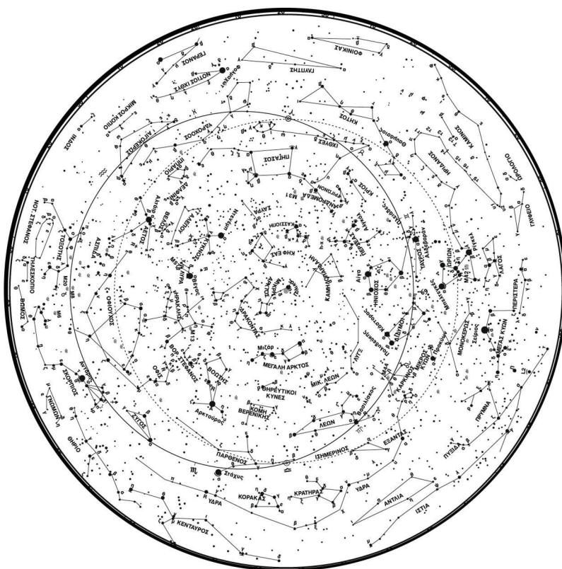
Εικόνα 2: Χάρτης του ουρανού με τους αστερισμούς του βορείου ημισφαιρίου. Επεξεργασία εικόνας: Ελβίρα Μεταλληνού.
